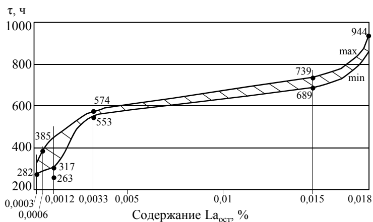
Рис. 1. Влияние остаточного содержания лантана на долговечность \tau сплава ВЖМ4-ВИ при испытании на длительную прочность при 1100^{\circ}\text{C} , \sigma=137 МПа
