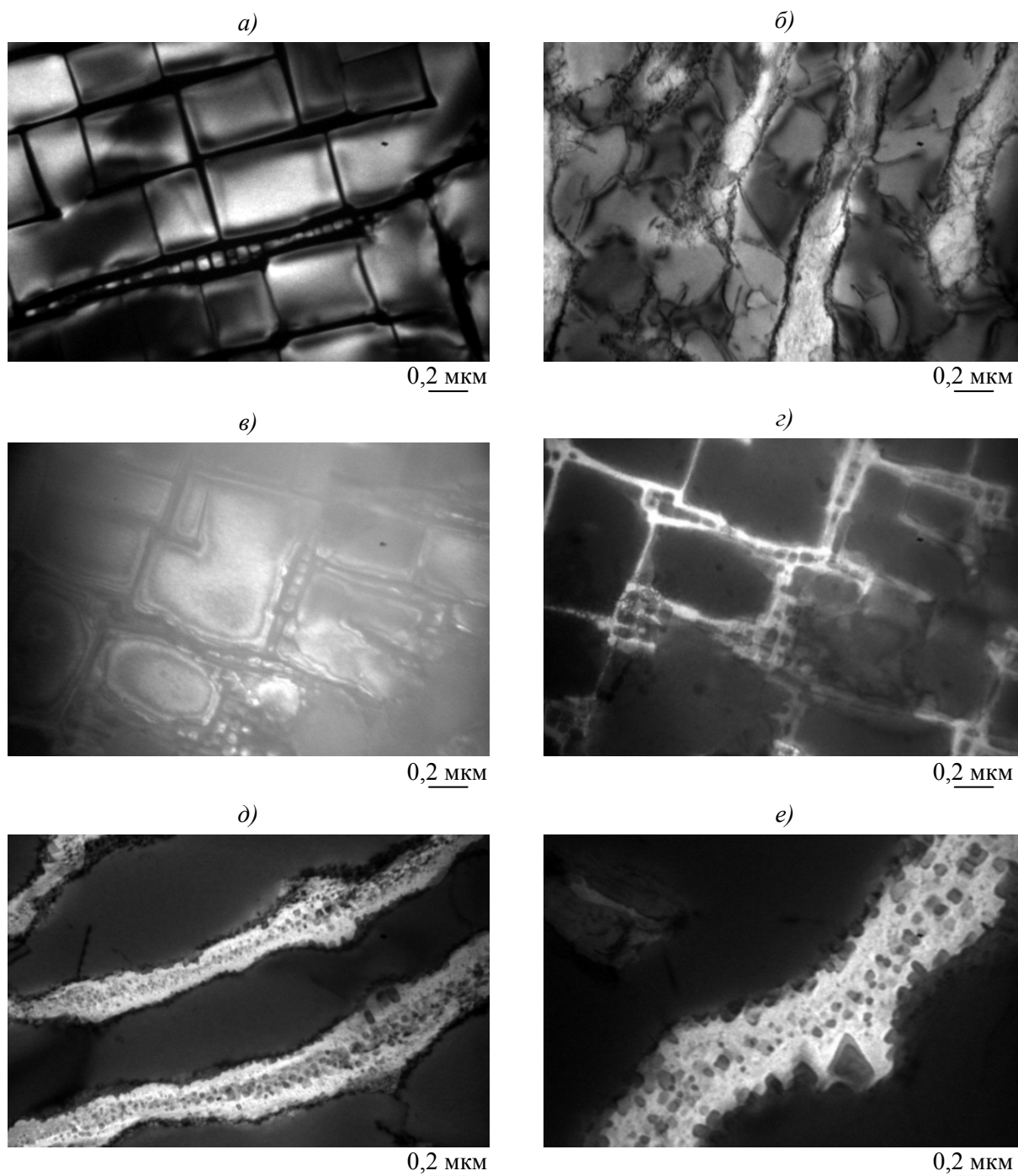
Рис. 2. Микроструктуры монокристалла (исследование на просвечивающем электронном микроскопе) из сплава ВЖМ4-ВИ без лантана ( a, б ) и с 0,015% \text{La}_{\text{ост}} ( в-е ) после полной термической обработки ( a, в, г ) и испытаний на длительную прочность при 1100°C, \sigma=137 МПа в течение 282 ( б ) и 739 ч ( д, е )
