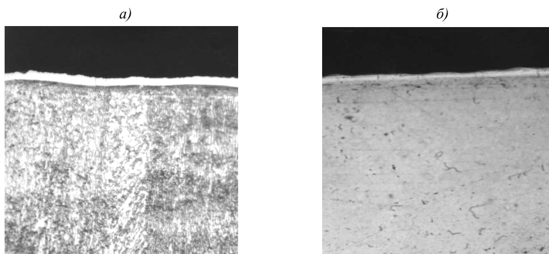
Рис. 3. Микроструктура ( \times 500 ) образцов с модифицированными слоями: а – основа – титановый сплав ВТ8М-1, осаждение в плазме Ni-Cr-Al-Y; б – основа – титановый сплав ВТ9, модифицирование в плазме Ni-Cr-Al-Y
