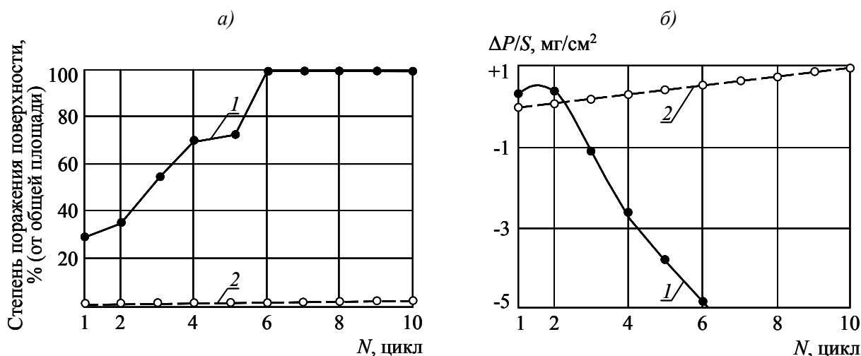
Рис. 5. Коррозионная стойкость (а – степень поражения поверхности; б – потери (привес) массы) стали ЭИ961 при циклических испытаниях (1 цикл: нагрев при 600°C, 1 ч → охлаждение до 20°C в 3%-ном растворе NaCl → выдержка во влажной атмосфере 22 ч):
