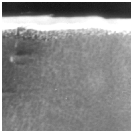
Рис. 4. Микроструктура ( \times 600 ) образцов стали ЭИ961 после ионного модифицирования в плазме сплава системы Al–Co–Si–Y
