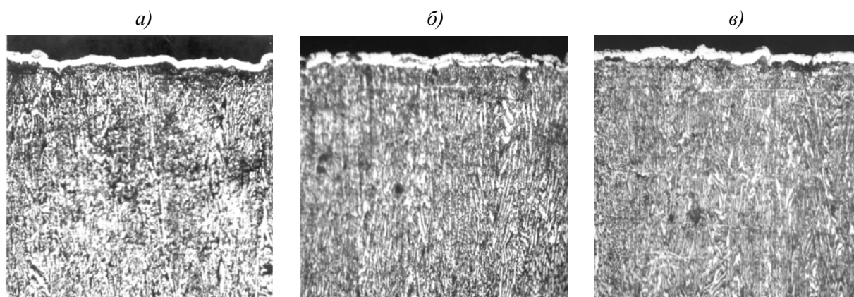
Рис. 8. Микроструктуры образцов из сплава ВТ8М-1 после ионного модифицирования в плазме сплава Ni-Al-Y:
