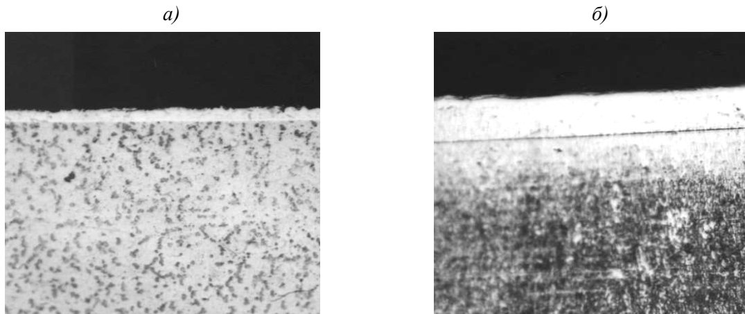
Рис. 2. Микроструктура ( \times 500 ) образцов с модифицированными слоями: a – основа – титановый сплав BT8M-1, осаждение в плазме Ni–Al–Y; б – основа – титановый сплав BT8M-1, модифицирование в плазме Ni–Al–Y
