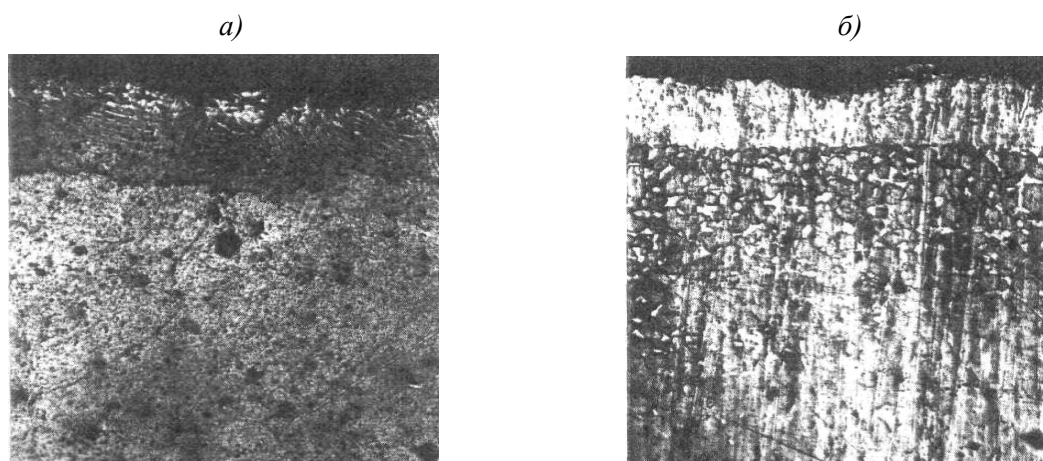
Рис. 1. Микроструктура ( \times 500 ) образцов с модифицированными слоями: a – основа – титановый сплав ВТ18У, модифицирование в плазме Zr–Y; б – основа – сталь ЭП866, модифицирование в плазме Ti
