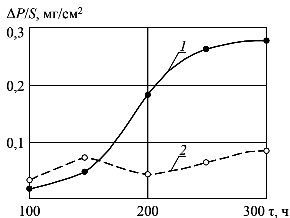
Рис. 6. Жаростойкость стали ЭИ961 при 600°C:
