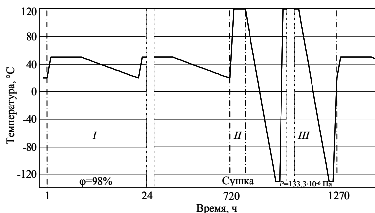
Рис. 2. Схема ускоренных испытаний конструктивных панелей:
